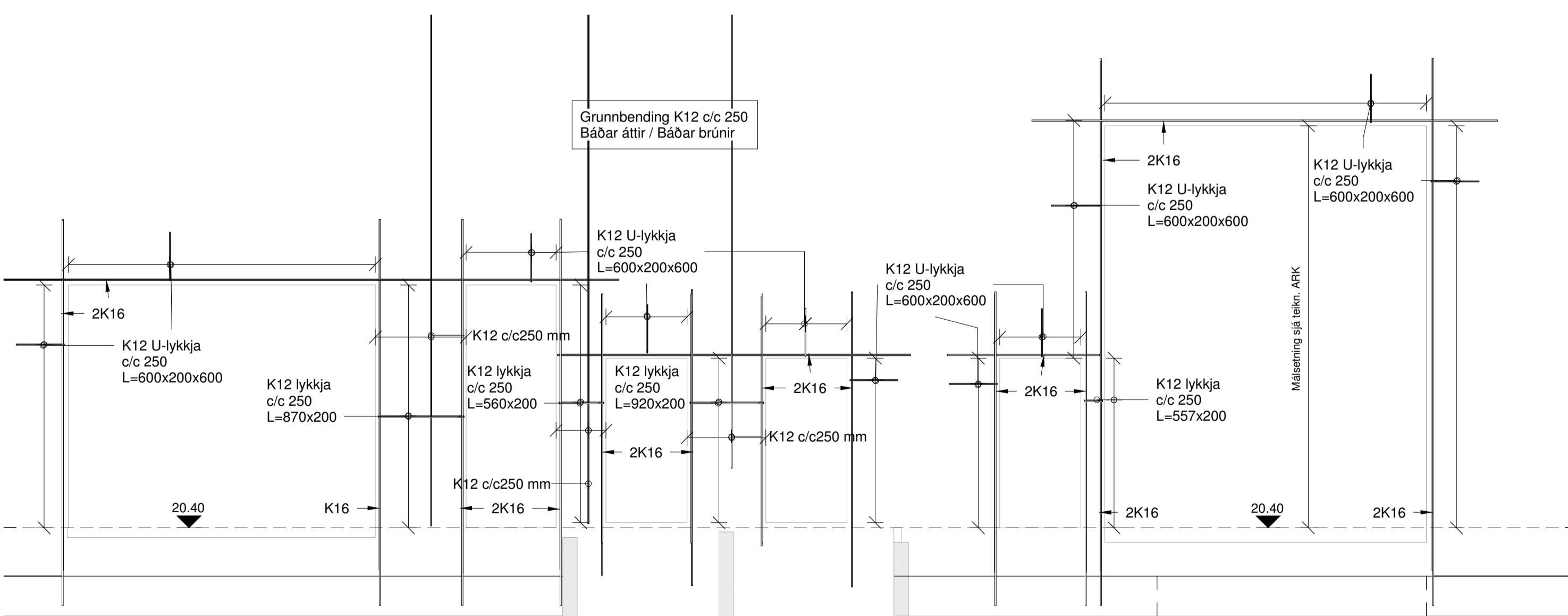
BG SNID B2 011 1 : 50
