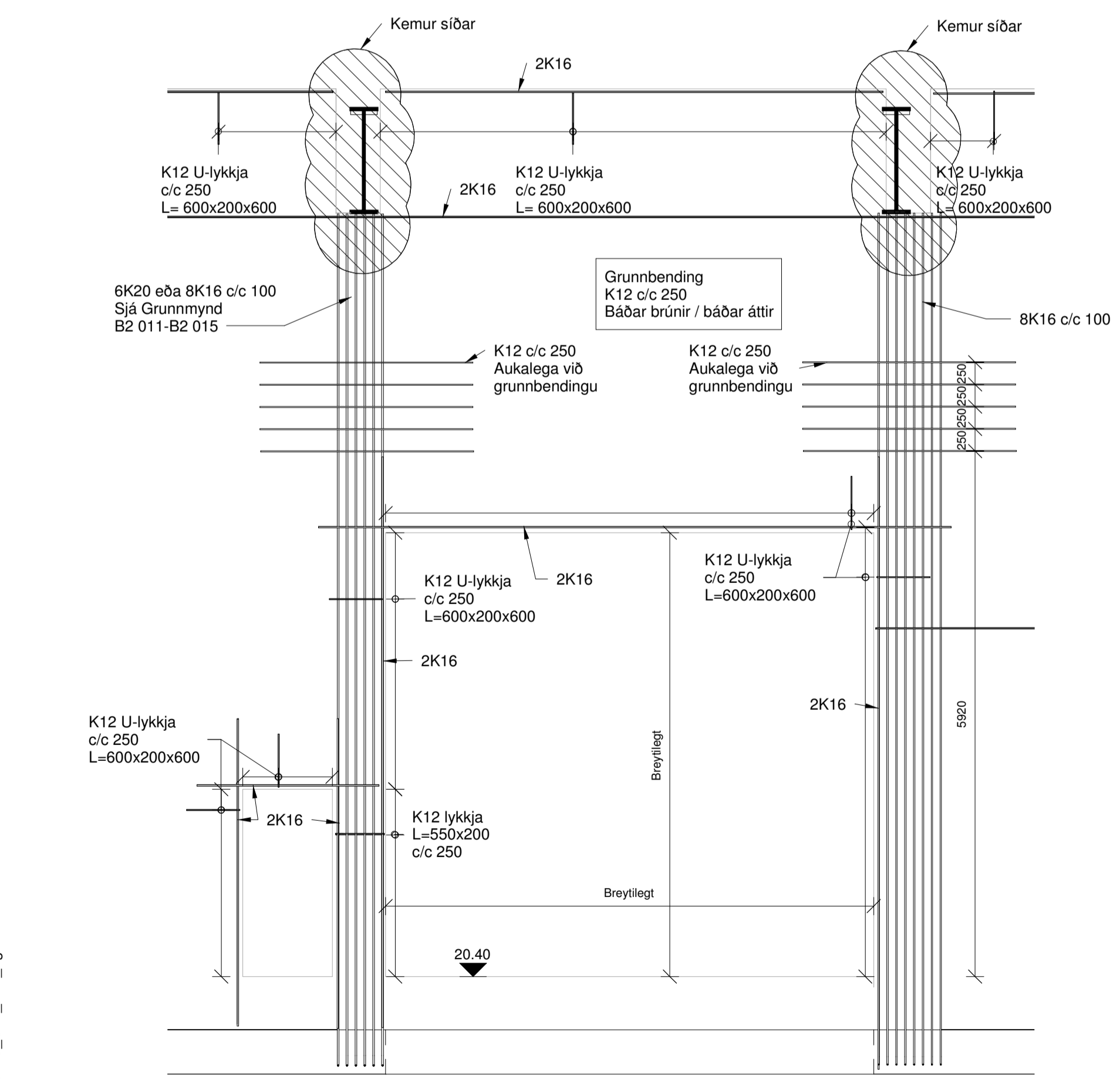
BA SNID B2 011 1 : 50
