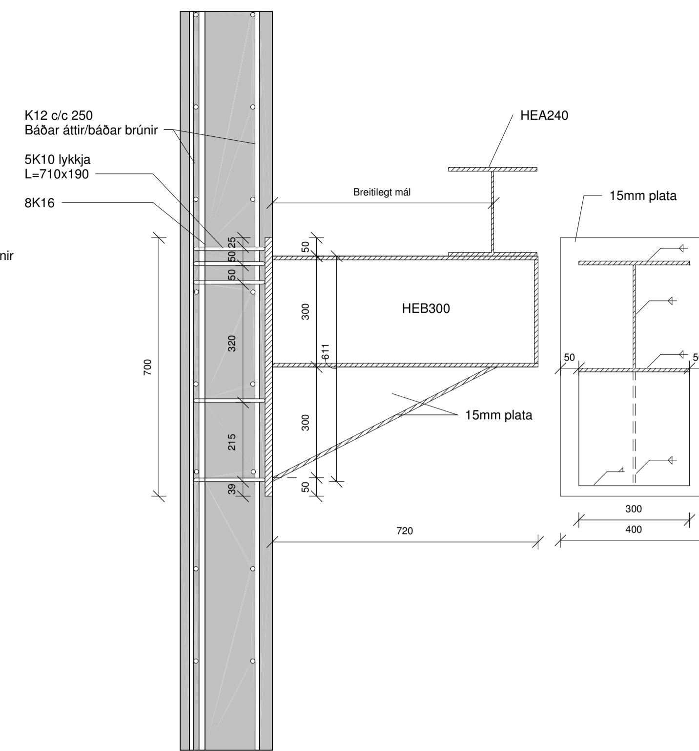
BJ SNID B2 011 1 : 50
