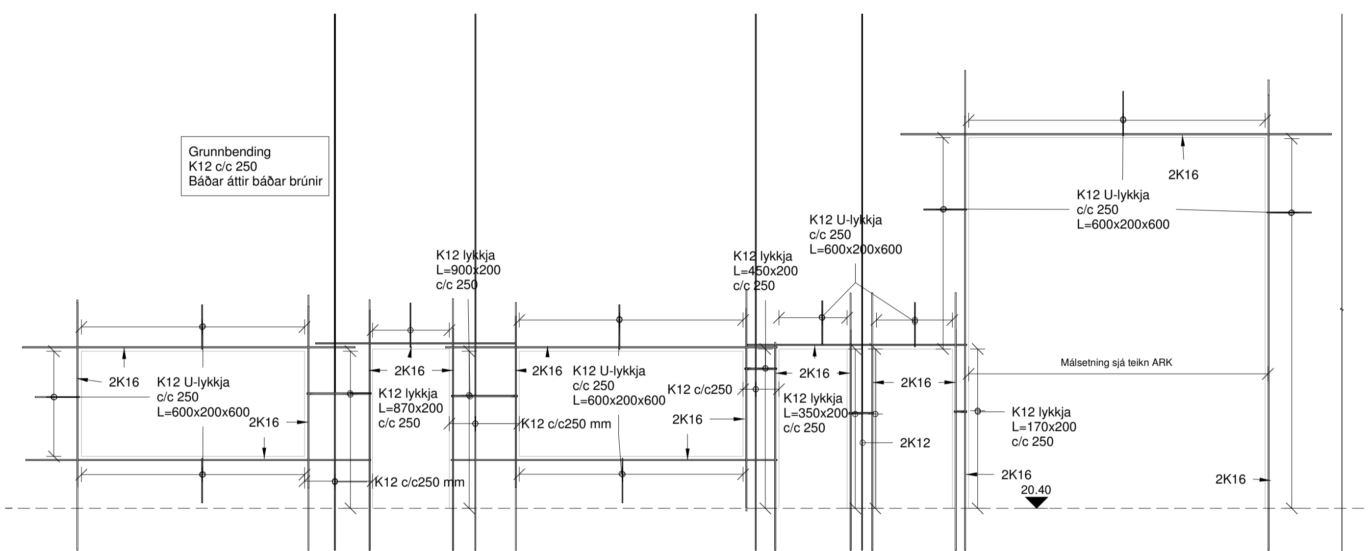
BE SNID B2 015 1 : 50
