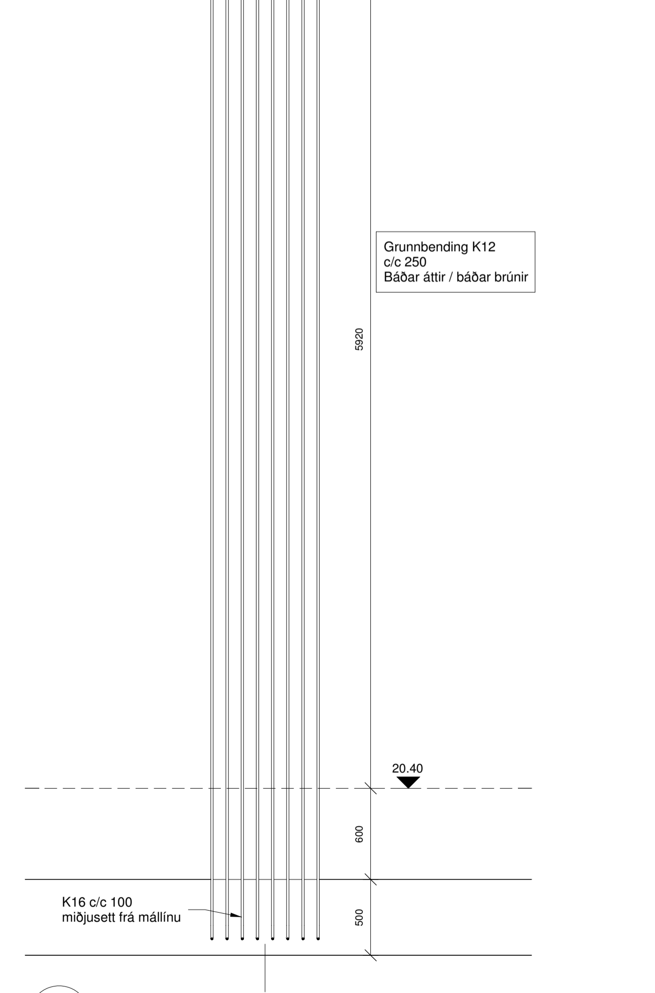
BB SNID B2 011 1 : 25
