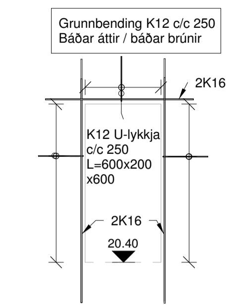
BF SNID B2 011 1 : 50
