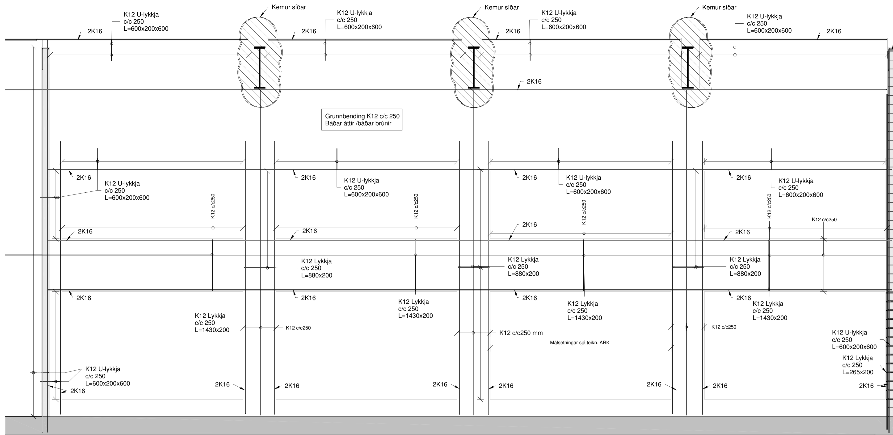
BA SNID B2 011 1 : 50
