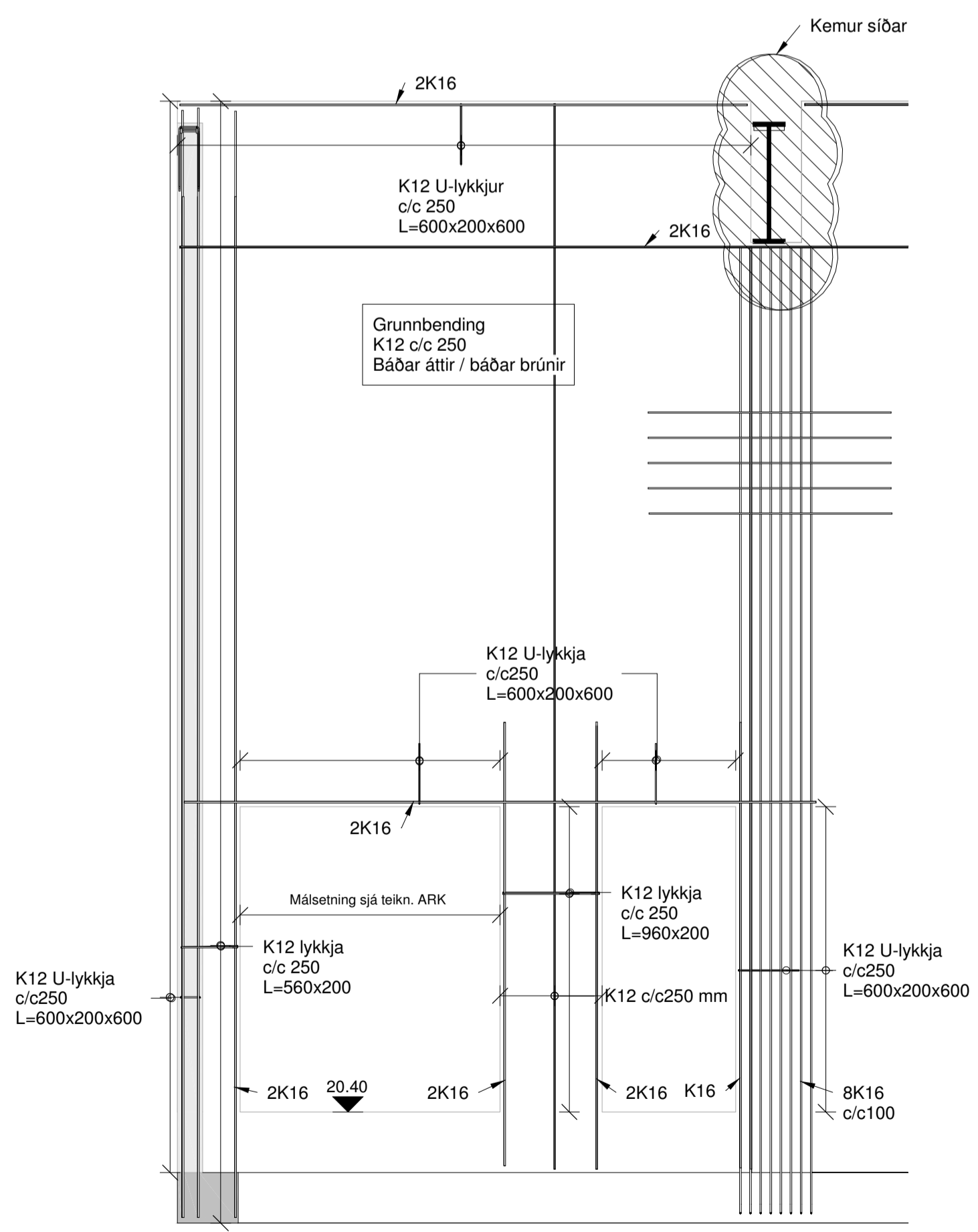
BD SNID B2 015 1 : 50
