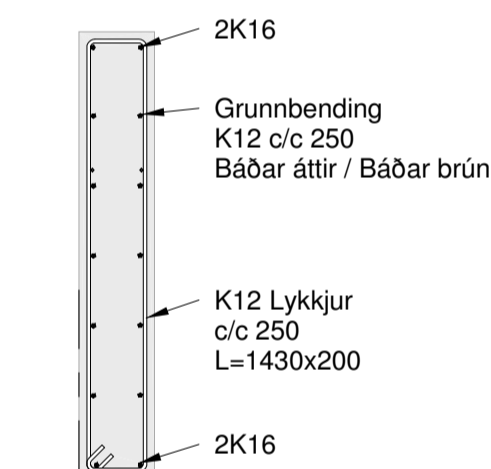
BI SNID B2 011 1 : 25
