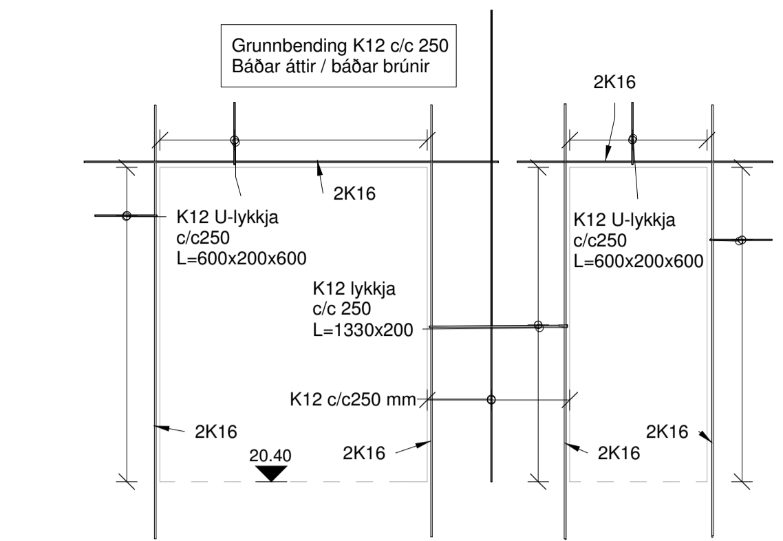
BE SNID B2 015 1 : 50
